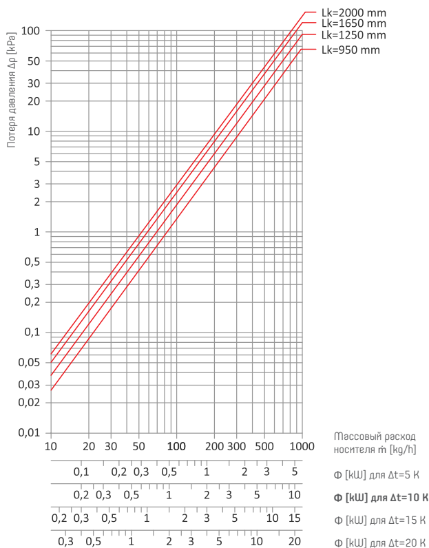
VKN1-6,5/14/Lk VKN1-9/14/Lk
